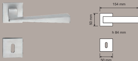
486 RB 024 | Maniglia con rosetta ribassata art.024 / Door handle on reduced rose art.024
