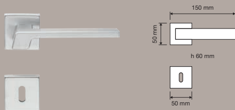
484 RB 088 | Maniglia con rosetta art.088 / Door handle on rose art.088
