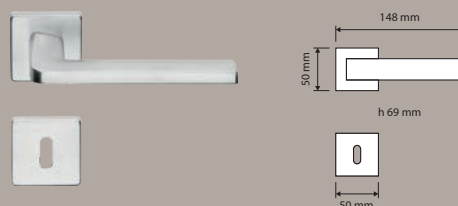
419 RB 088 | Maniglia con rosetta art.088 / Door handle on rose art.088
