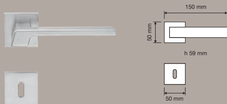
484 RB 024 | Maniglia con rosetta ribassata art.024 / Door handle on reduced rose art.024
