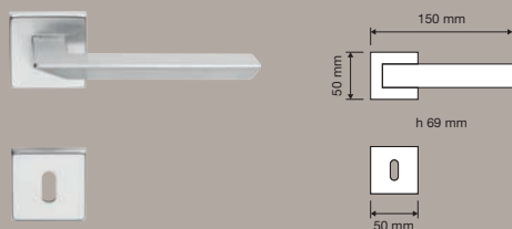
485 RB 088 | Maniglia con rosetta art.088 / Door handle on rose art.088
