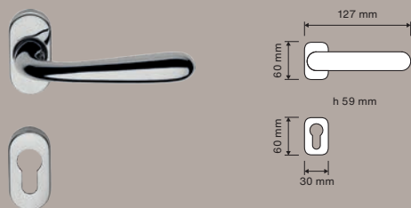
498 RB 096 | Maniglia con rosetta art.096 / Door handle on rose art.096
