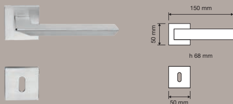
485 RB 024 | Maniglia con rosetta ribassata art.024 / Door handle on reduced rose art.024
