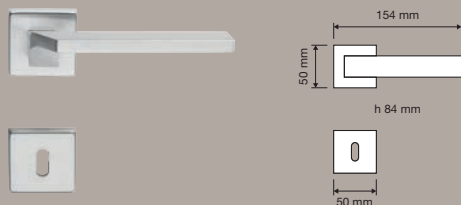
464 PL | Maniglia con placca art.475 / Door handle on plate art.475
