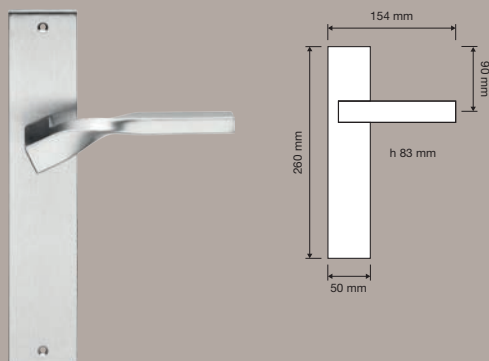
468 PL | Maniglia con placca art.475 / Door handle on plate art.475
