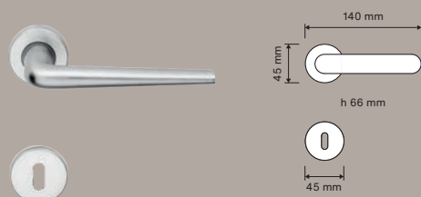
479 RB 101-45 | Maniglia con rosetta art.101 45 mm / Door handle on rose art.101-45 mm
