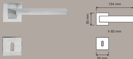
487 RB 024 | Maniglia con rosetta ribassata art.024 / Door handle on reduced rose art.024
