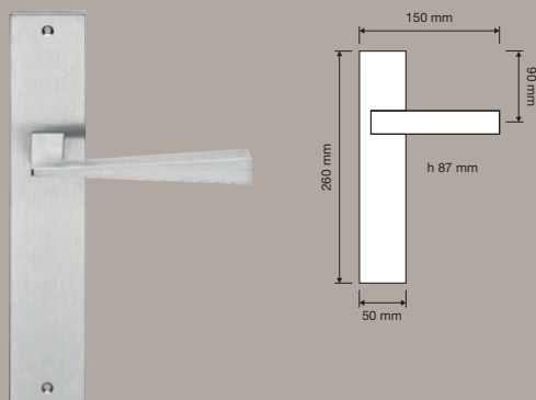
486 DK | Maniglia per finestra con movimento DK 4 posizioni / Window handle with DK movement 4 clicks
