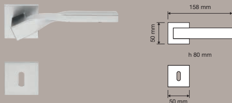
489 RB 024 | Maniglia con rosetta ribassata art.024 / Door handle on reduced rose art.024
