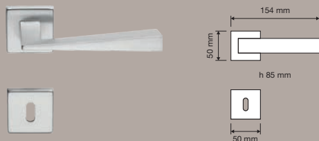
486 RB 088 | Maniglia con rosetta art.088 / Door handle on rose art.088
