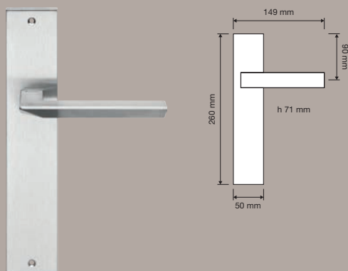
465 PL | Maniglia con placca art.475 / Door handle on plate art.475
