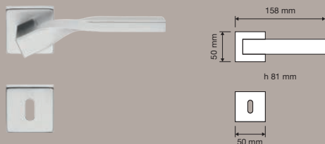
489 RB 088 | Maniglia con rosetta art.088 / Door handle on rose art.088
