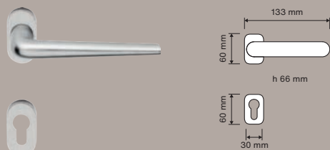
479 RB 096 | Maniglia con rosetta art.096 / Door handle on rose art.096
