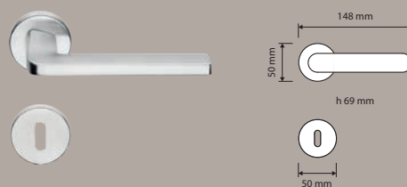
419 RB 027 | Maniglia con rosetta art.027 / Door handle on rose art.027
