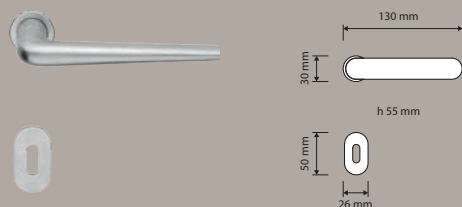
479 RB 085 | Maniglia con rosetta autoadesiva art.085 senza molla / Door handle on self-adhesive rose art.085 without spring
