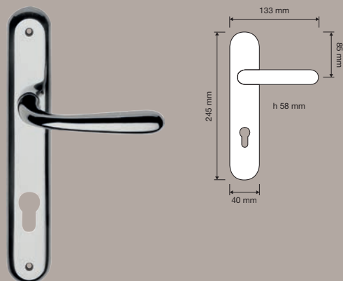
498 PL | Maniglia con placca art.670 / Door handle on plate art.670
