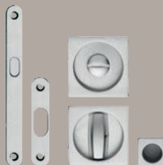
196 KT | Kit incasso quadro con placche piene e maniglia trascinamento / Square inset handle blind hole kit with finger pull
