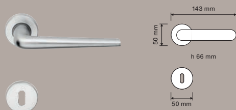
479 RB 101-50 | Maniglia con rosetta art.101 50 mm / Door handle on rose art.101-50 mm
