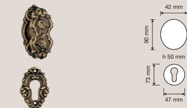
1210 PG 075 Pomolo a girare con rosetta art.075 / Turnable knob on rose art.075
